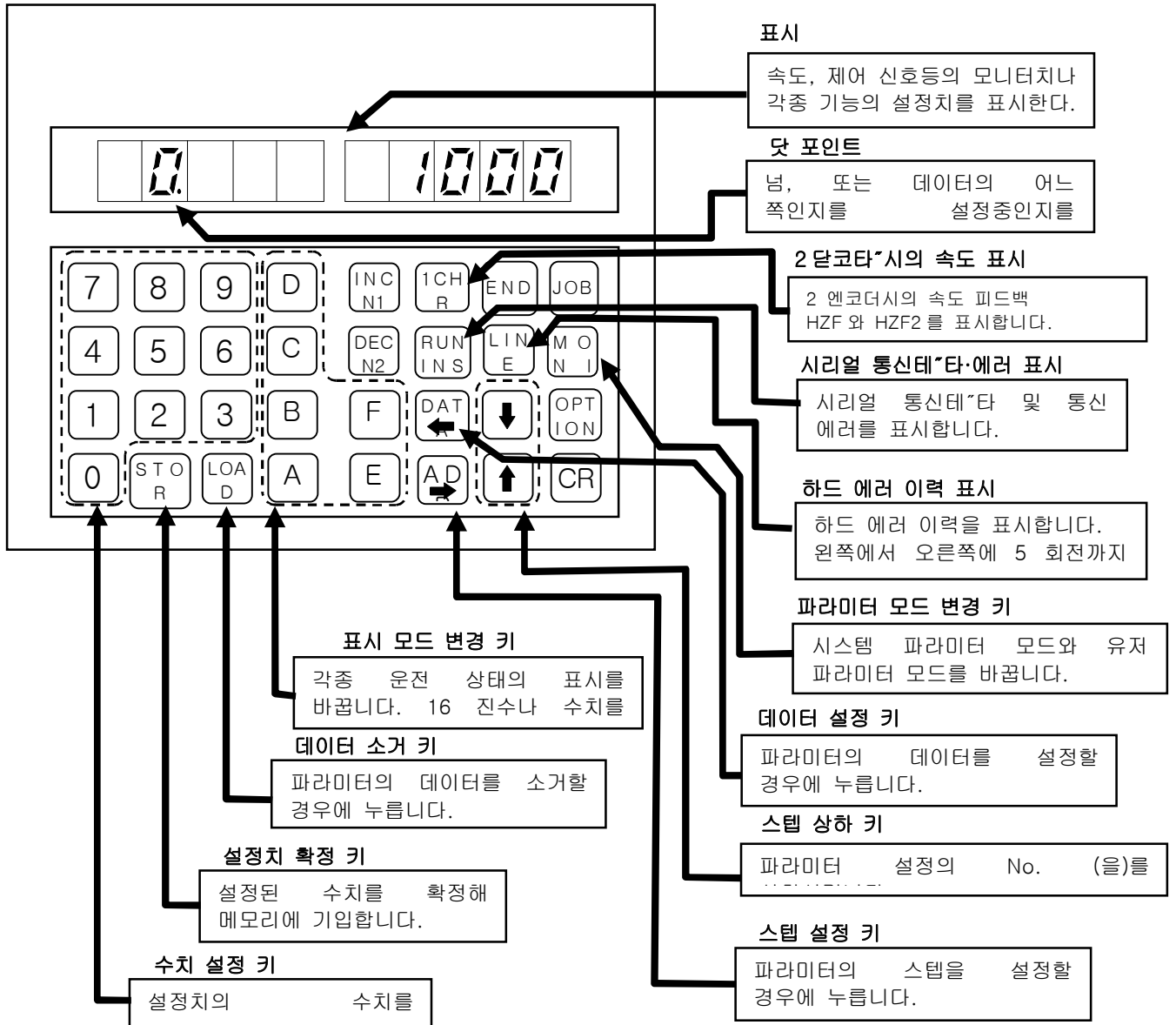
그림 11-1 키보드·디스플레이의 배치
