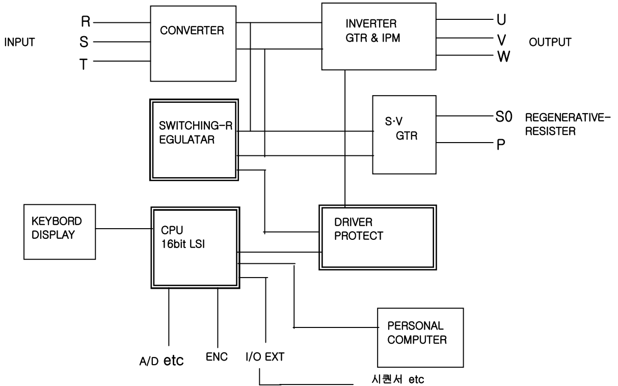
제 7-1 도 MS-SERVO 구성도
